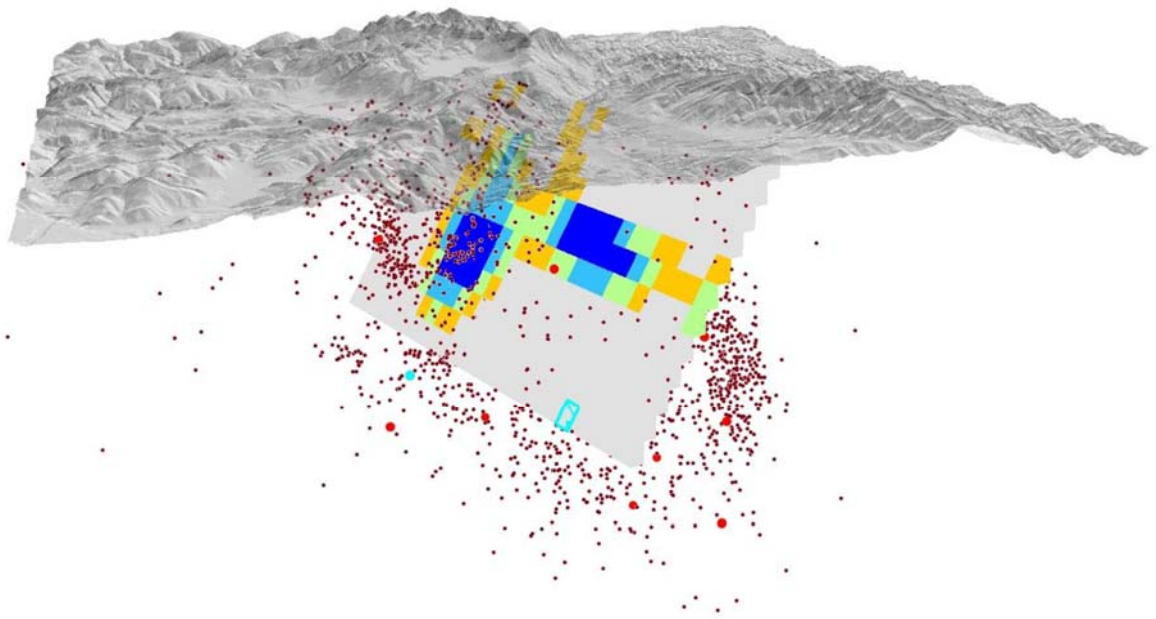
Fig. 5 - Preliminary 3D view of the seismogenic fault obtained by inversion of the static ground displacement (2 datasets SAR and 3 CGPS; Gruppo di Lavoro INGV sul terremoto di Amatrice, 2016).
