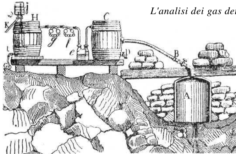
Apparecchio del Payen per la raccolta dei gas dei soffioni.
